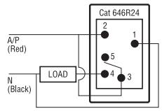
646R24 Timer
