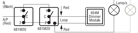
625F/625FM Fan Speed Control
